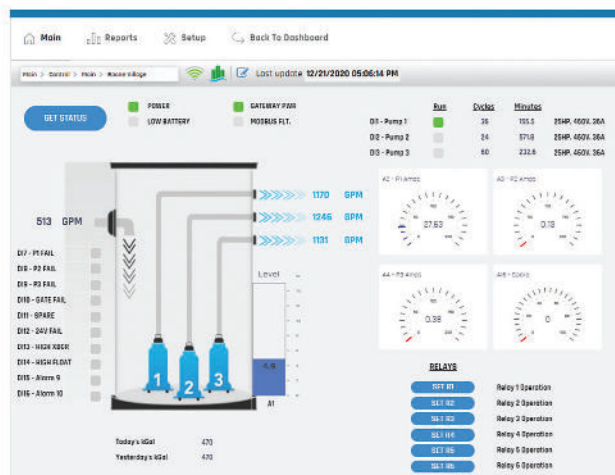
Estación de Bombeo (Duplex / Triplex)
