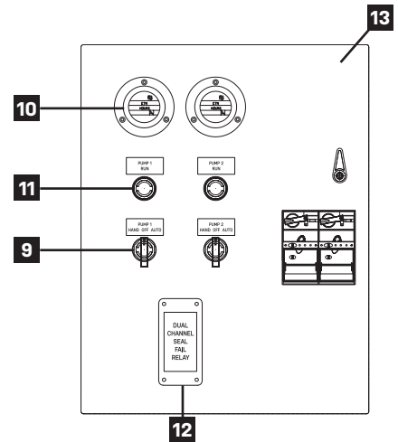
Inner Door
